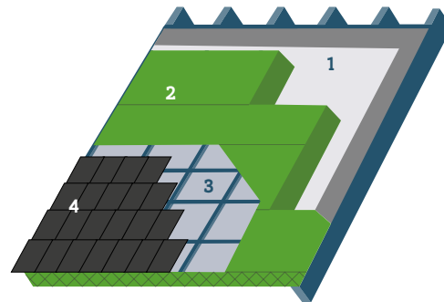
1. Dampschermbekleding 2. Isolatie 3. Onderdak 4. Dakbekleding
