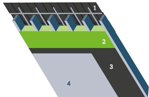
1. Onderdak 2. Isolatie 3. Dampschermbekleding 4. Binnenafwerking
